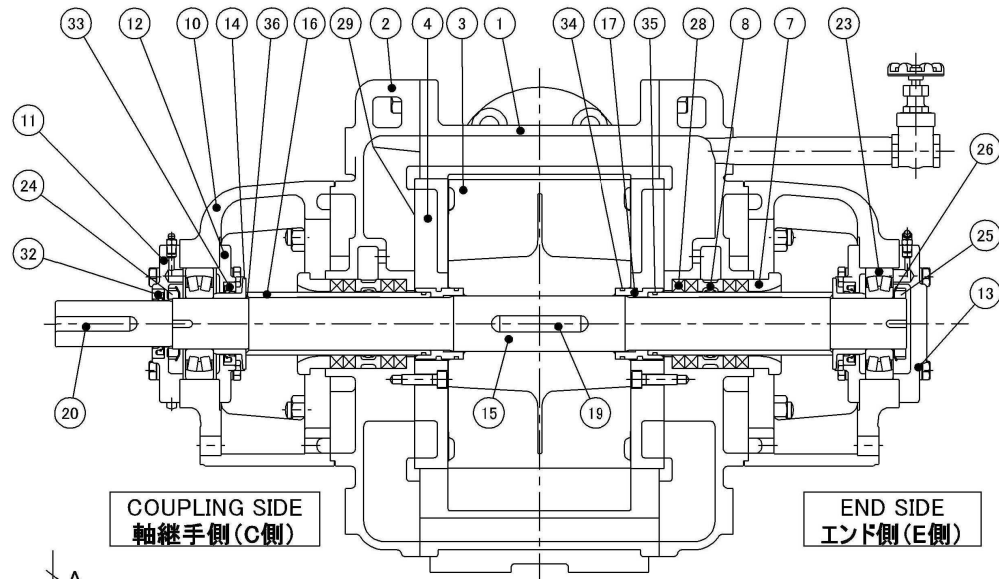
断面図 A-A
