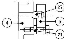
DETAIL OF BALL VALVE ボールバルブ詳細
